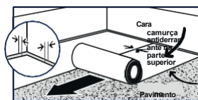
JUNTA DE DILATAÇÃO PERIMETRAL
